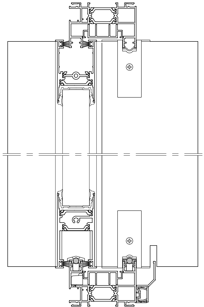
COUPE VERTICALE
